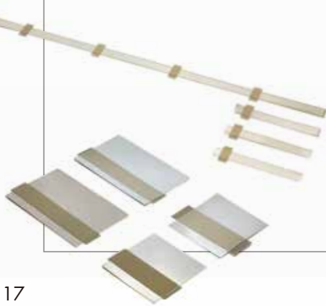
极耳
